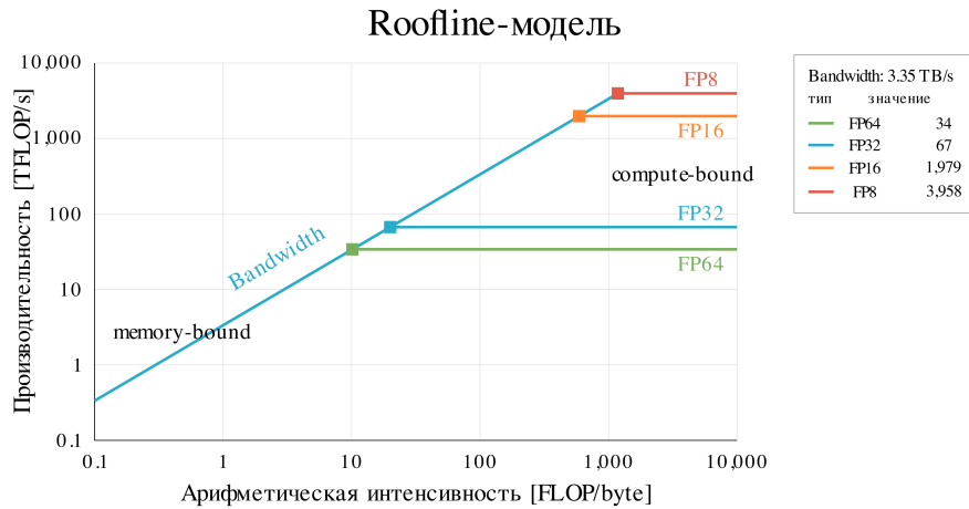
Рис. 17: Roofline-модель.
